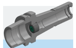
Sensore Balluff interno
